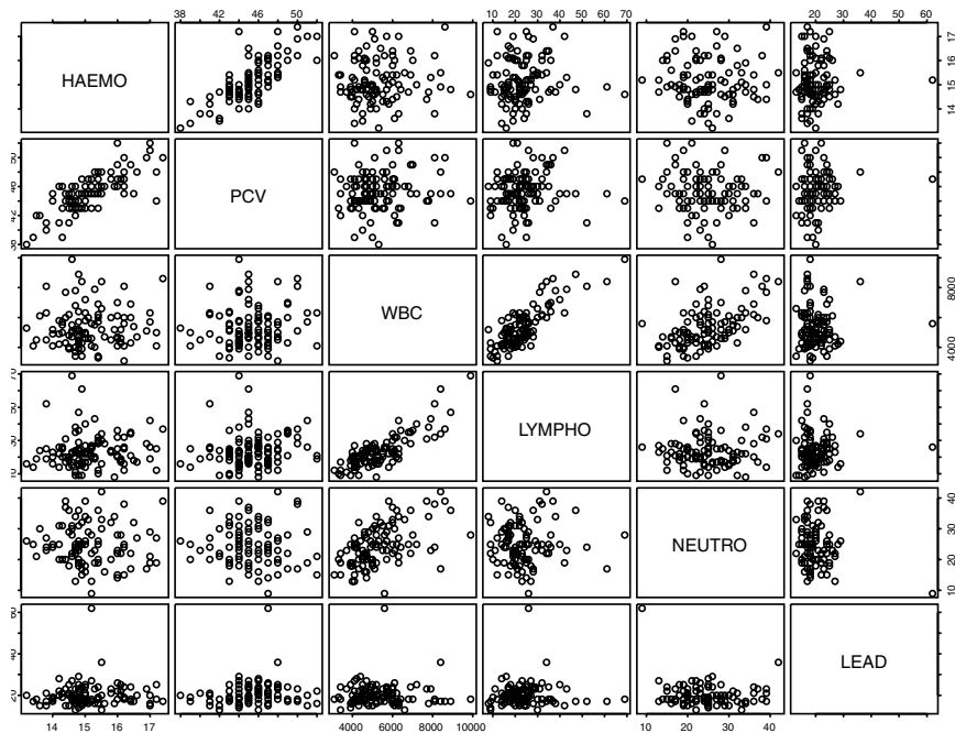
Fig. 59 Draughtsman’s plot.
